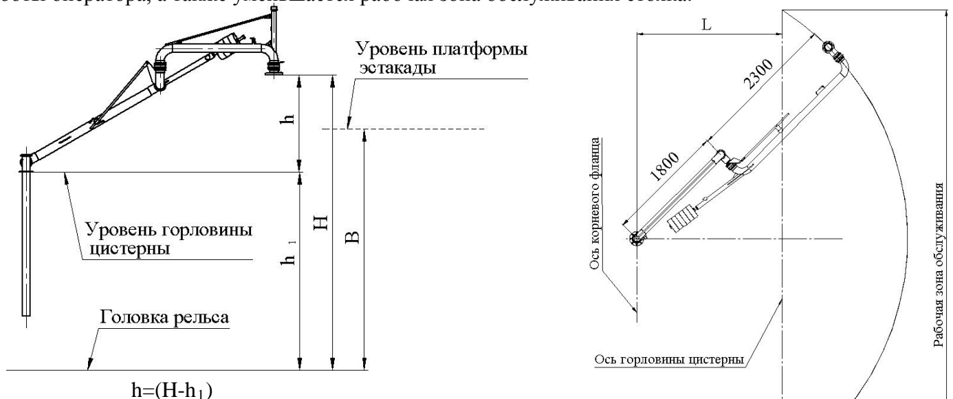
Рис. 2. Рабочая зона обслуживания стояка ОСН-СВН-100-Н-А-6-НН.
