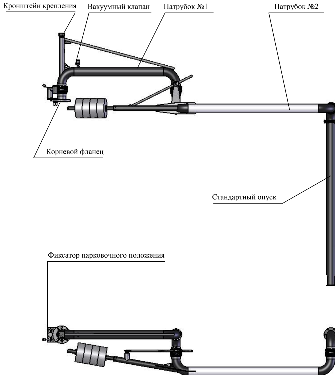
Рис. 1. Конструкция стойки верхнего налива ОСН-СВН-100-Н-А-6-НН.
